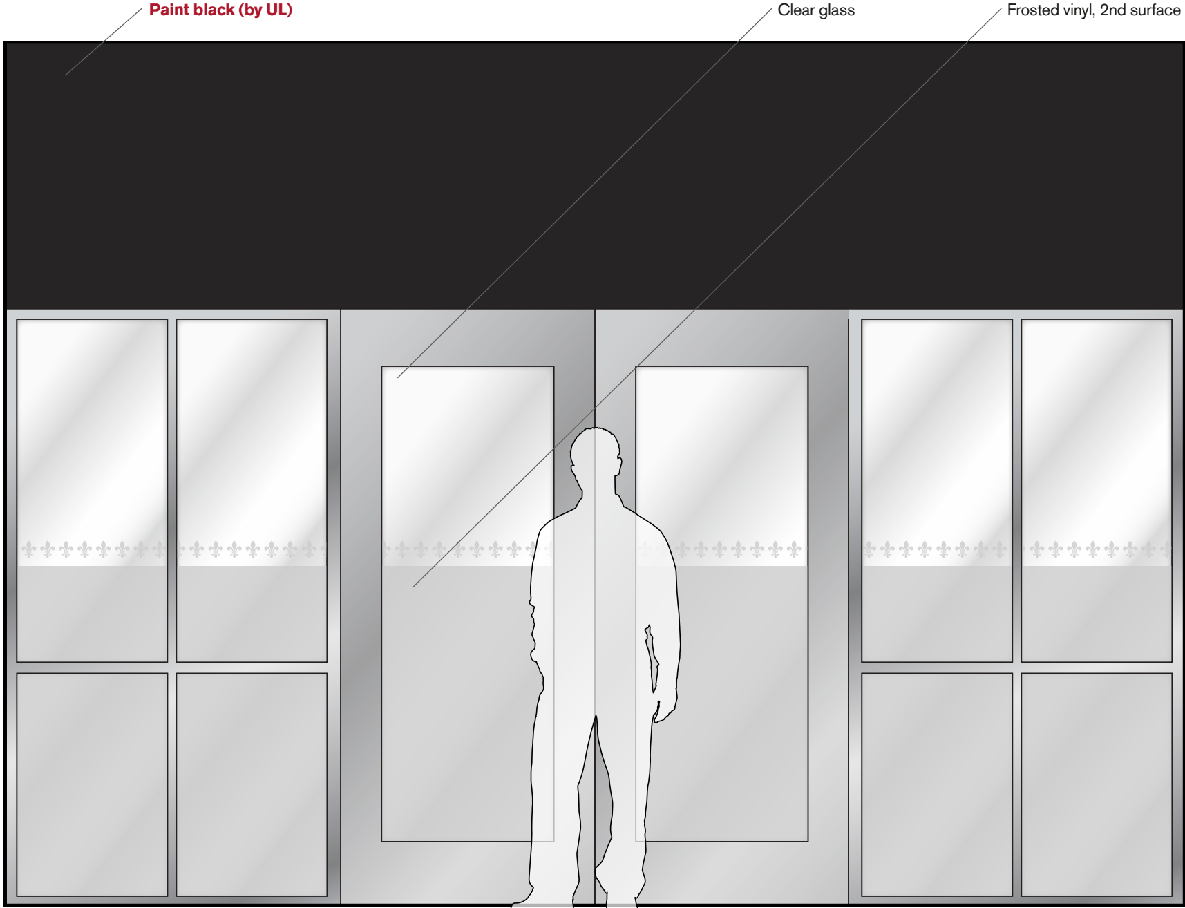
ELEVATION // EAST
